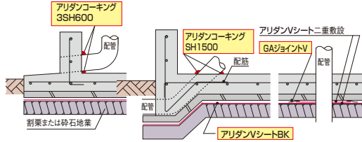
参考納まり図
