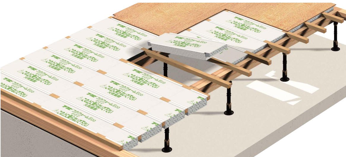
根太間用納まり
