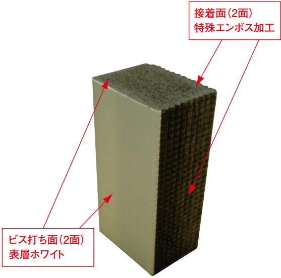
寸法:30×40(L=78mm) 1袋=500個入(包装形態:PP不織布袋)
