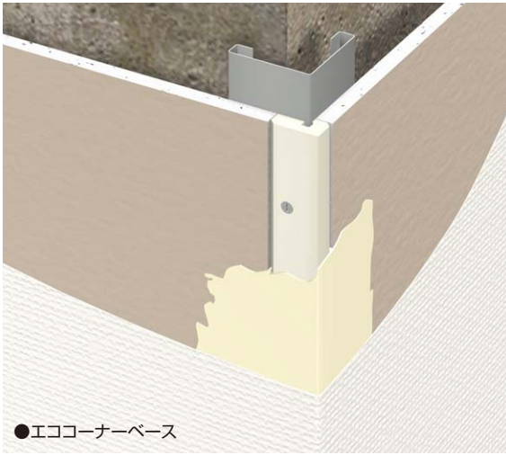
参考納まり図
