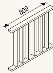
縦格子パネル W900
