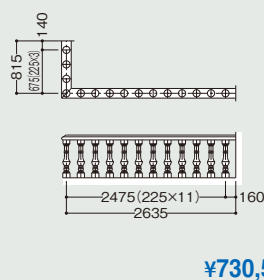
●手摺ET02 / 手摺子BA04
