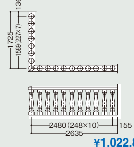
●手摺ET01 / 手摺子BA05
