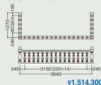
●手摺ET02 / 手摺子BA04 / 親柱BG00
