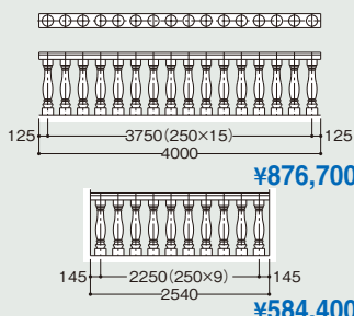
●手摺ET01 / 手摺子BA05
