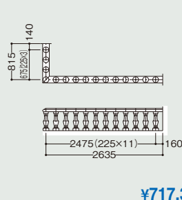
●手摺ET02 / 手摺子BA06
