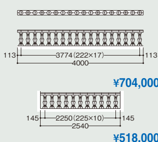
●手摺ET02 / 手摺子BA06
