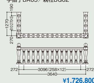
●手摺ET01 / 手摺子BA05 / 親柱BG02
