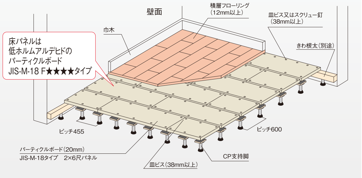
CP支持脚 遮音タイプ
