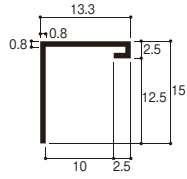
●スッキリ見切10
