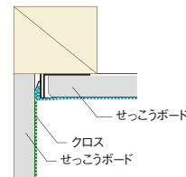
参考納まり図
