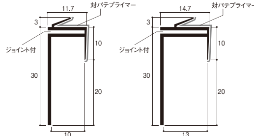
●先付けクロスフリー見切10
