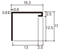
●スッキリ見切13
