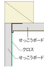
参考納まり図
