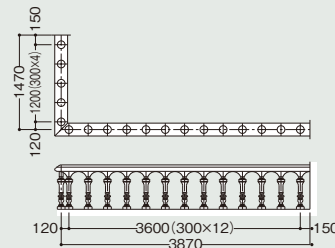
●手摺ET01 / 手摺子BA01
