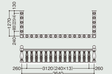
●手摺ET02 / 手摺子BA02 / 親柱BG00
