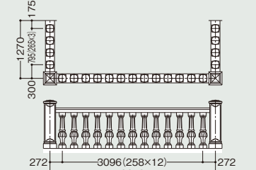
●手摺ET01 / 手摺子BA03 / 親柱BG01
