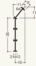
3 コーナー定木C型 製品図
