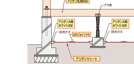
参考納まり図
