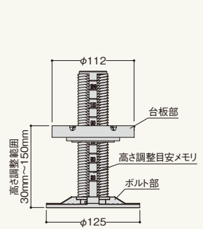
■マルチポストBC型 製品図
