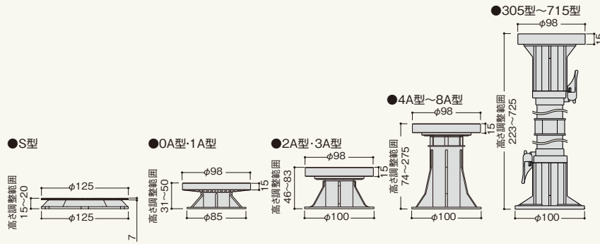
■マルチポスト 製品図
