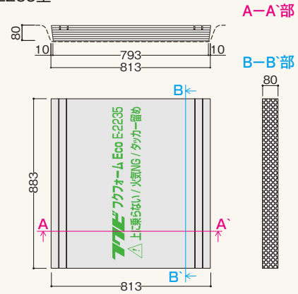
2 E-2235型
