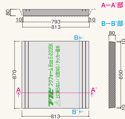
5 E-2235K型
