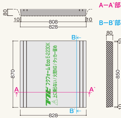
4 E-2230K型
