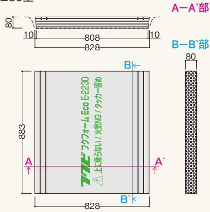
1 E-2230型
