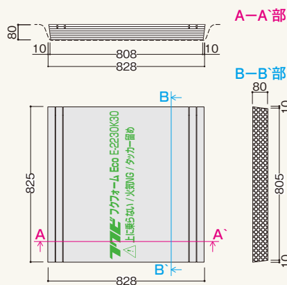
6 E-2230K30型
