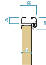
プラス棒付き外枠寸法
