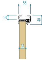
プラス棒付き外枠寸法
